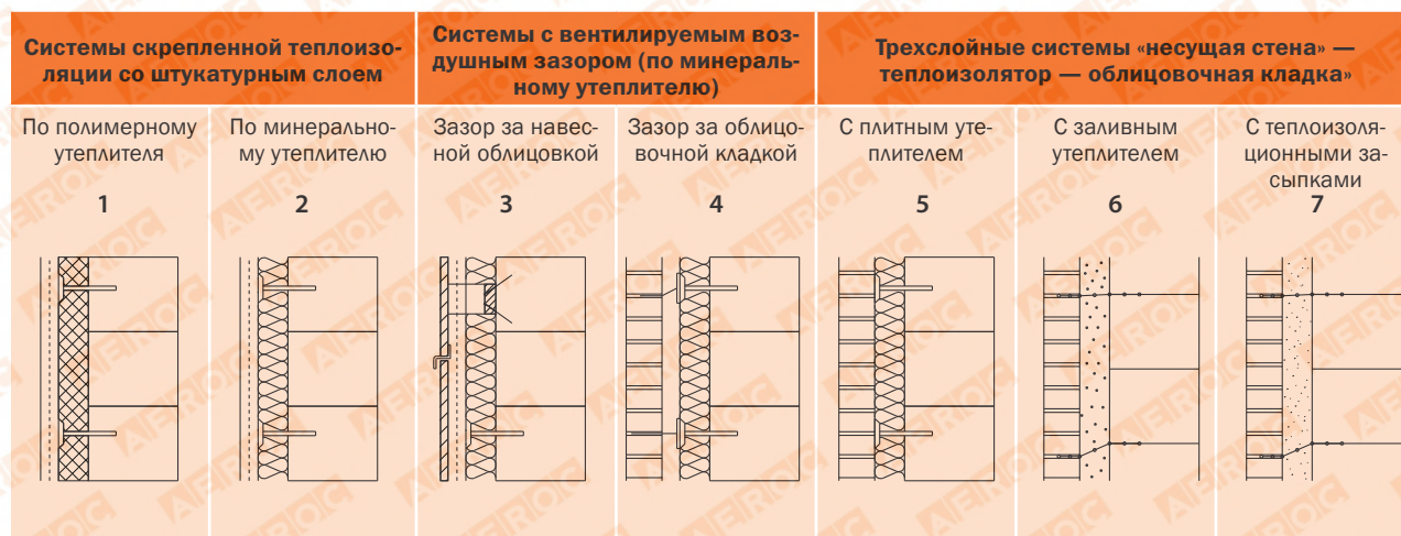
Рис. 18. Системы теплоизоляции.
