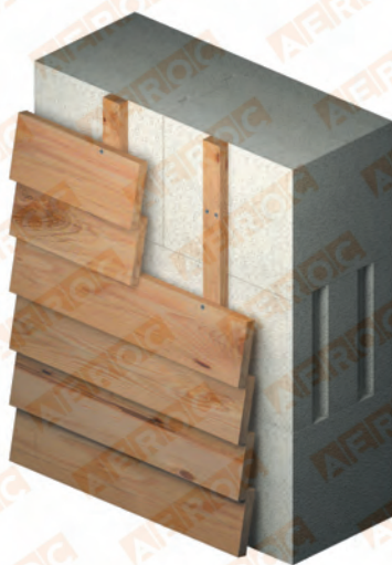
Рис. 7а. Облицовка по направляющим
