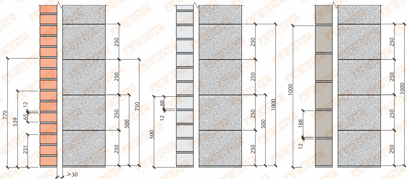
А - облицовка одинарным кирпичем. Высота ряда 65+12=77 мм.
