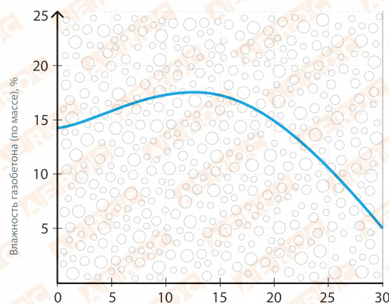
Рис. 5. Влияние дождей и штукатурки на влажность газобетона (стена из D400 через полгода после кладки).
