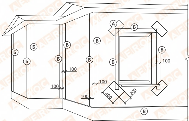
А – углы проемов. Сетка 200х400 мм Б – углы кладки, ребра откосов. Угловой профиль и сетка. Наклест сетки по 100 мм. Ширина полотна 100+100=200 мм В – примыкание к цоколю. Цокольный стартовый профиль.
