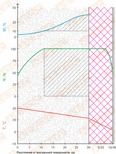
B2 – мокрое утепление по ППС 100 мм
