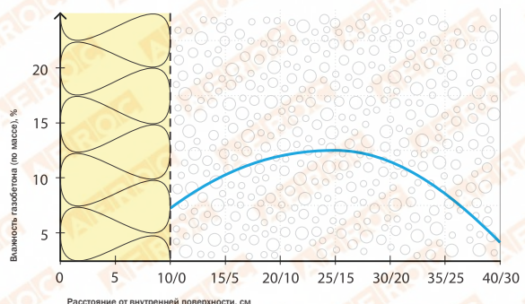
В - вентфасад по минвате
