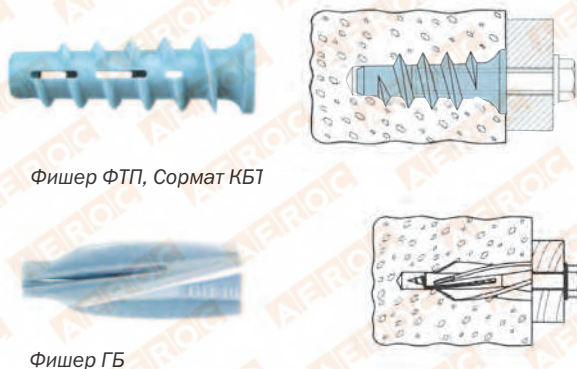
Рис. 11. Фотографии и схемы из каталога «Фишер. Крепежные системы»
