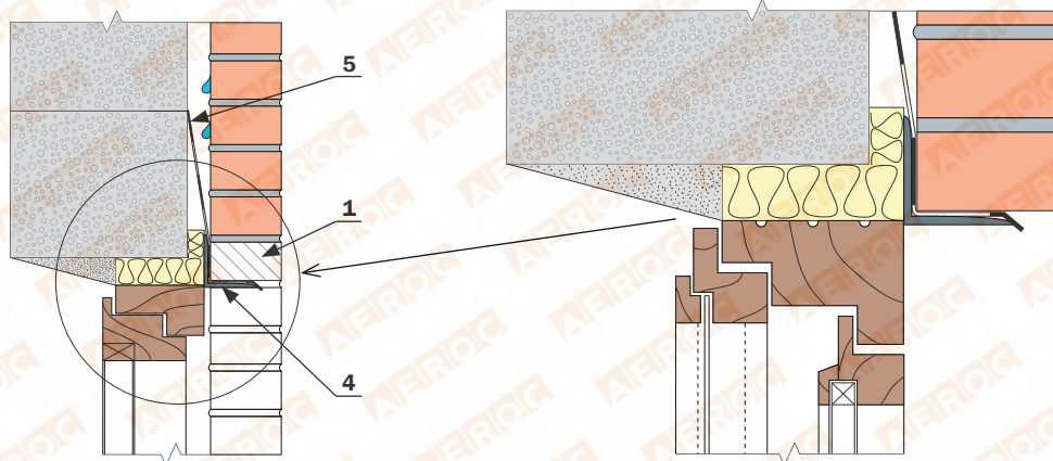
Б - над перемычкой.
