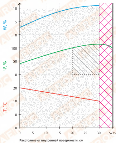
B1 – мокрое утепление по ППС 50 мм
