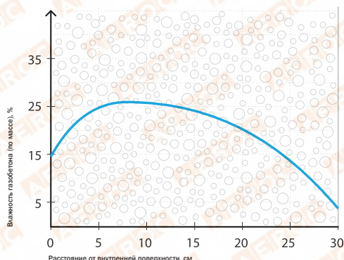
В - оштукатуренная кладка через 2 месяца после оштукатуривания
