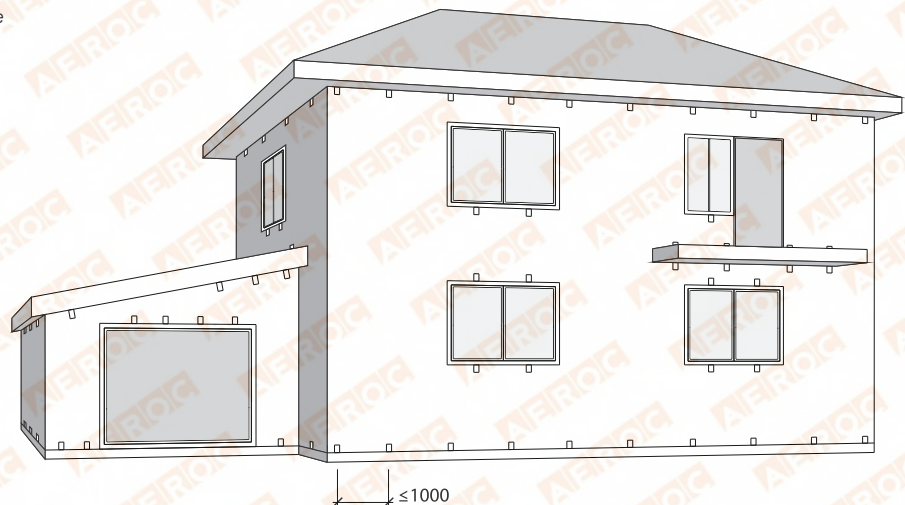
В - схема расположения вентиляционных и сливных отверстий.
