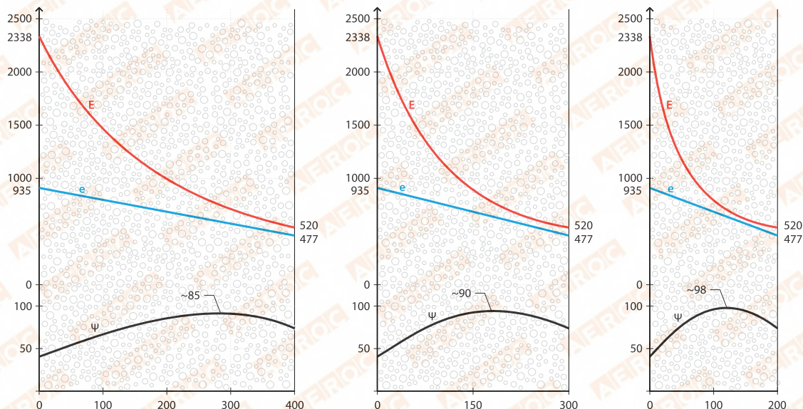
Рис. 25. Влияние толщины конструкции на распределение влажности воздуха в порах по толщине стены.
