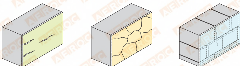
Рис. 17. Основные типы дефектов штукатурки.
