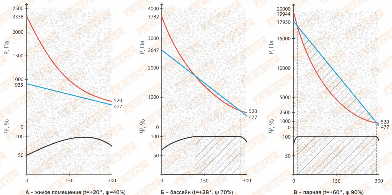
Рис. 24. Влияние микроклимата на распределение влажности воздуха в порах по толщине стены.
