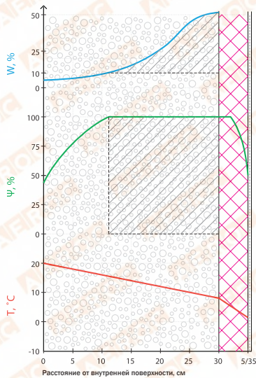
B1 – мокрое утепление по ППС 50 мм
