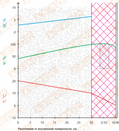
B3 – мокрое утепление по ППС 100 мм
