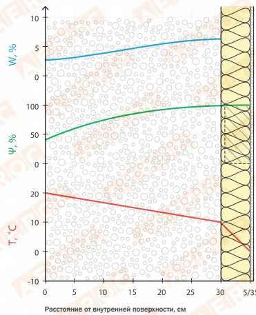
B2 – мокрое утепление по минвате 50 мм
