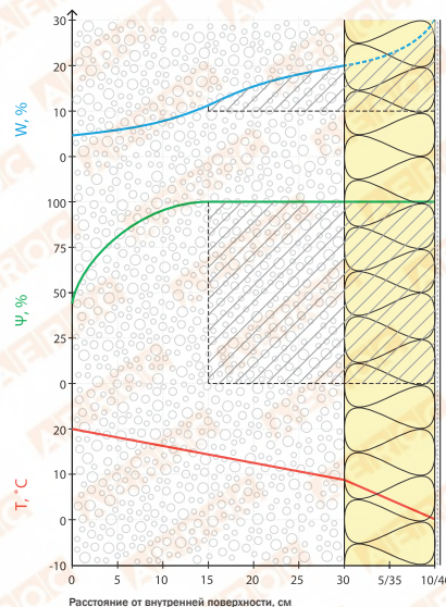
В2 – мокрое утепление по минвате 100 мм
