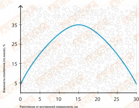
А - кладка через месяц после возведения
