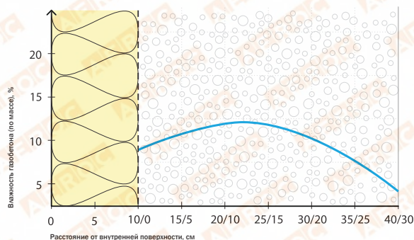
Б - штукатурка по минвате
